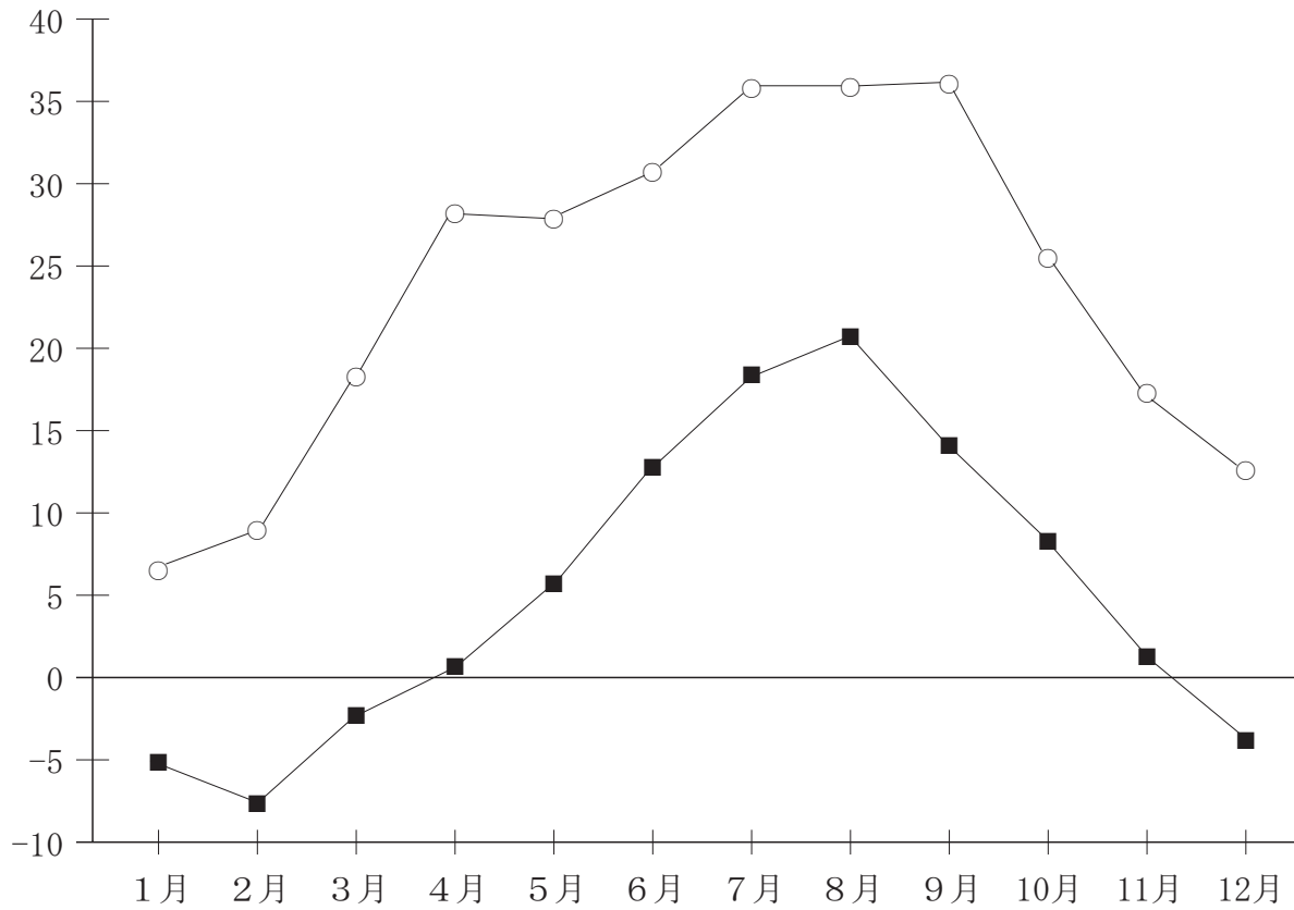
月別最高・最低気温（平成 24 年）
