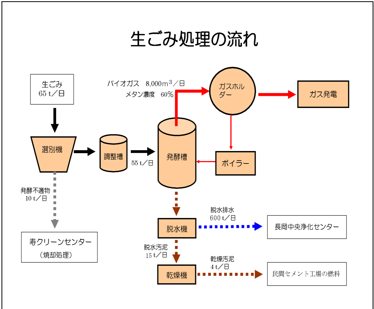
図 生ごみバイオガス化施設による生ごみ処理のイメージ
