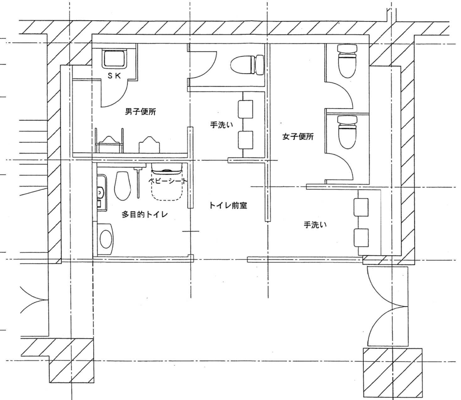
■ トイレ平面図
