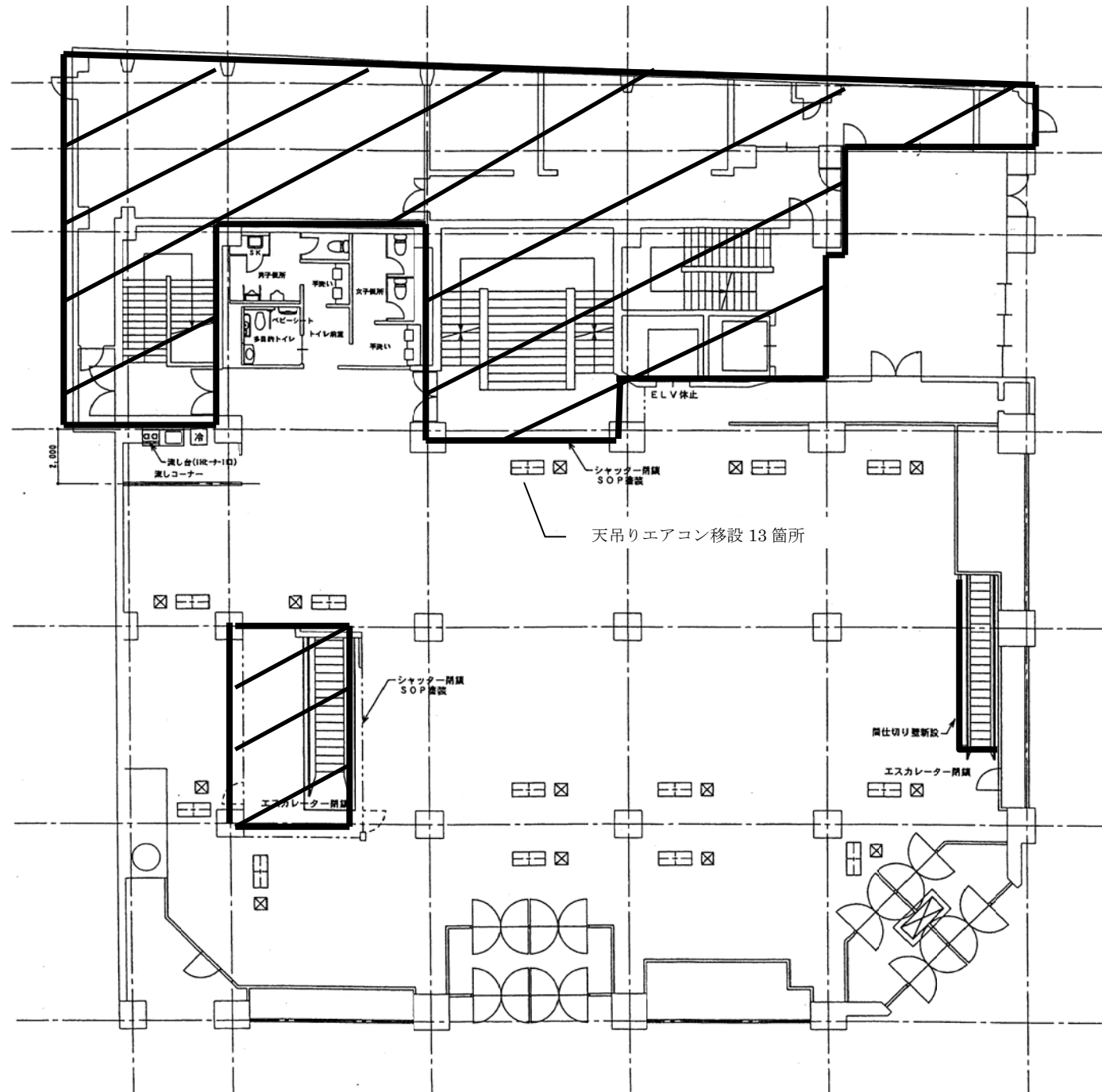
■ 1階平面図
