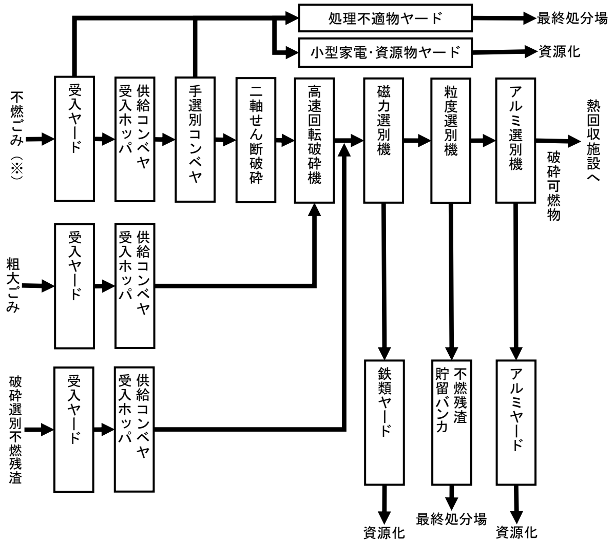
図 2 不燃・粗大ごみ処理施設処理フロー（参考）
