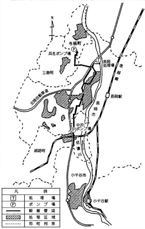
信濃川下流域下水道長岡処理区概要図
