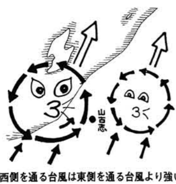
西側を通る台風は東側を通る台風より強い
