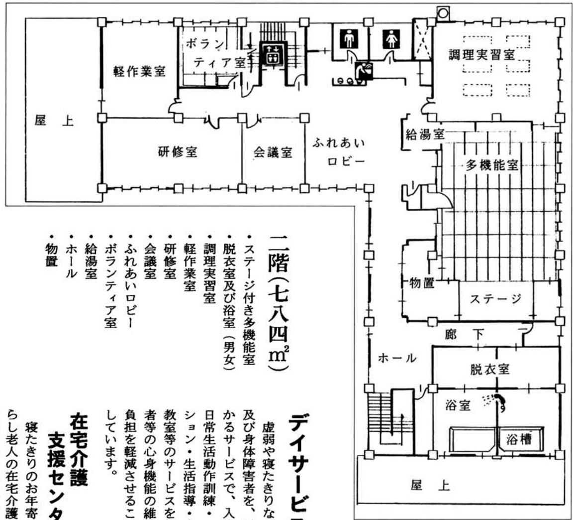
2階平面図
