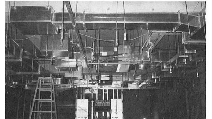
保健センター1F天井内配管ダクト機器吊込状況
