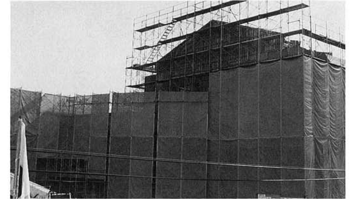
庁舎3F鉄筋・型枠組立状況
