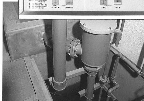
●自動荒目スクリーン 流入汚水中の砂および大きな浮遊物を取り除きます。 ●ばつ気沈砂槽
