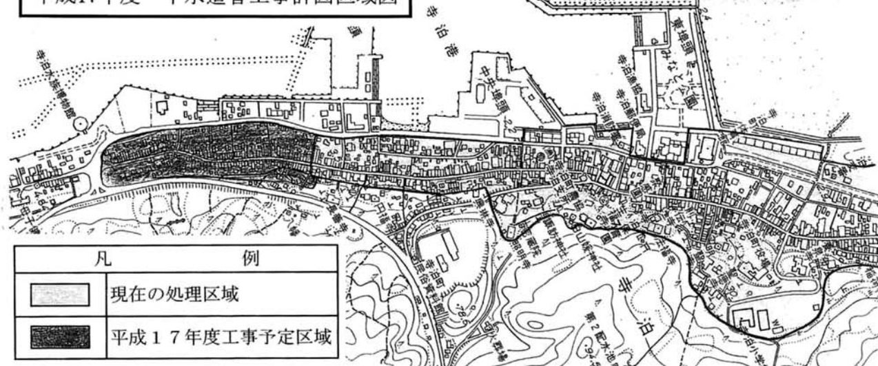
平成17年度 下水道管工事計画区域図
