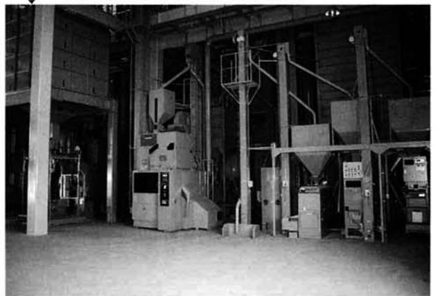
自主検査設備 ・各生産者毎のサンプルが乾燥され、検定装置で歩留測定をおこない検定データを精算事務へ引き継ぎます。
