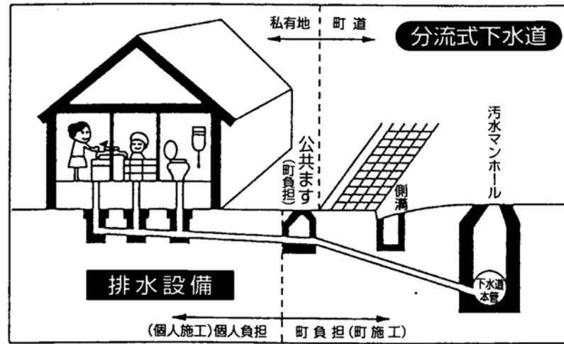
〈ます及び取付管の配置図〉
