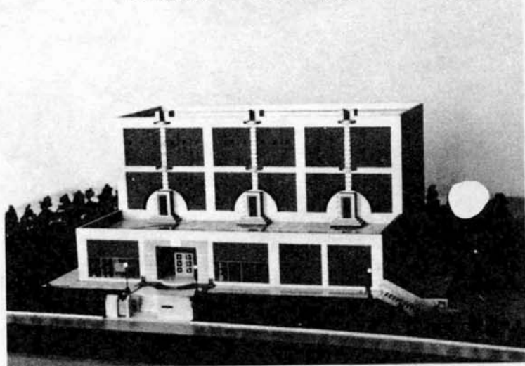
ごみ運搬用パイプライン集塵センター完成模型
