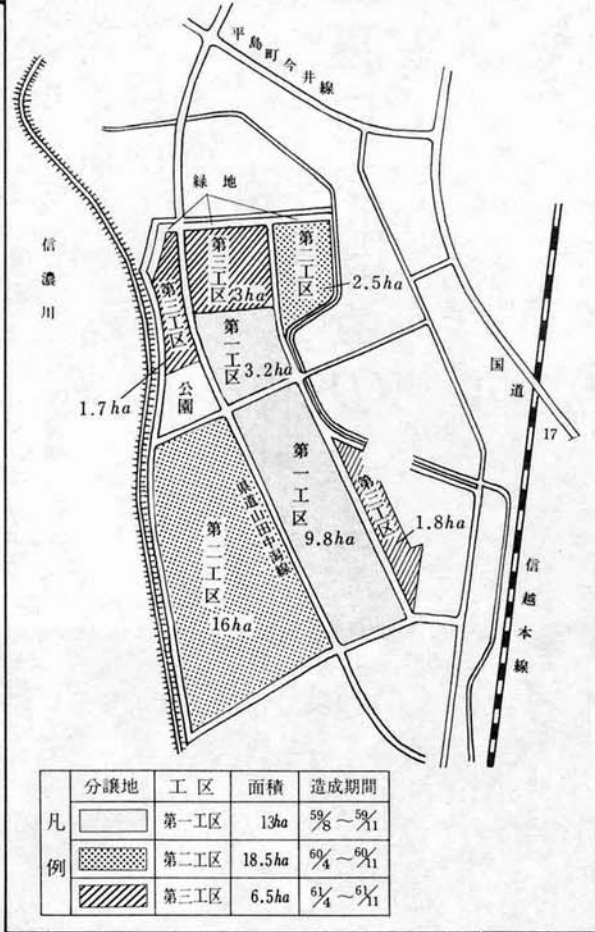
長岡市南部工業団地区区画図
