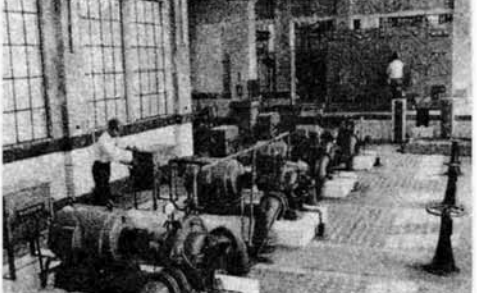
休みなく働く送水ポンプ……ここから市内に水を運び出します
