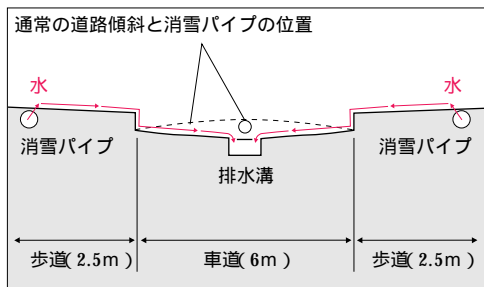
図1 歩道と車道の一体的な消雪を可能にした新しい道路構造
