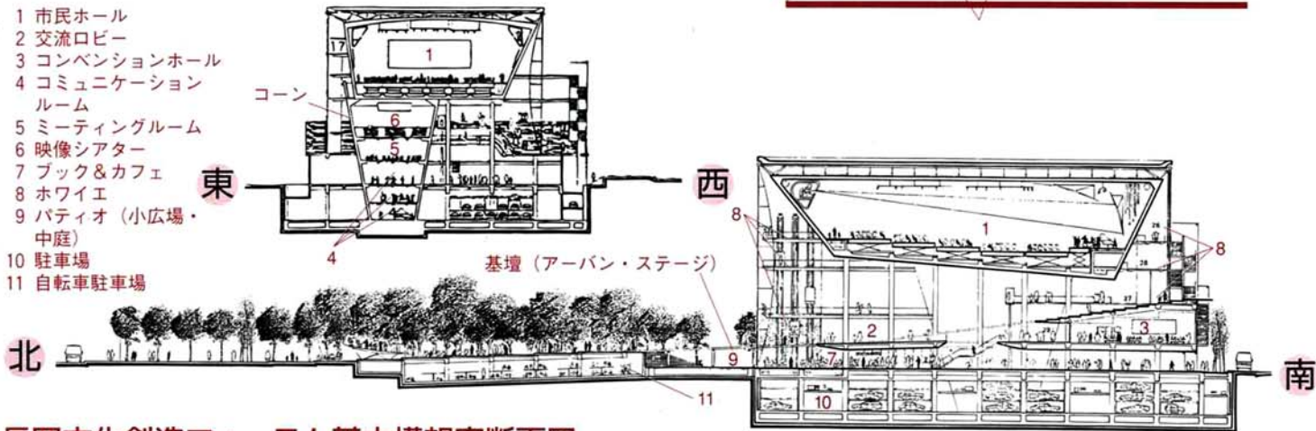
長岡文化創造フォーラム基本構想案断面図
