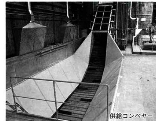
供給コンベヤーで運ばれたごみは破砕機の中で細かく砕かれ、鉄、アルミなど5種類に分別・処理されます
