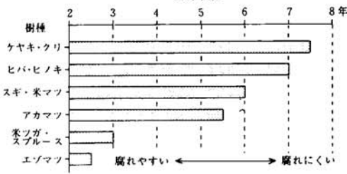
木材柱(3×3×60cm)を土壌中に半分差し込んで野外に放置したときの樹種別耐朽年数(心材)耐朽年数
