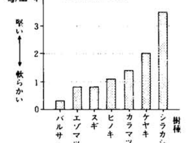
図-1 堅い木・軟らかい木(プリネル硬さ) 板目面での比較
