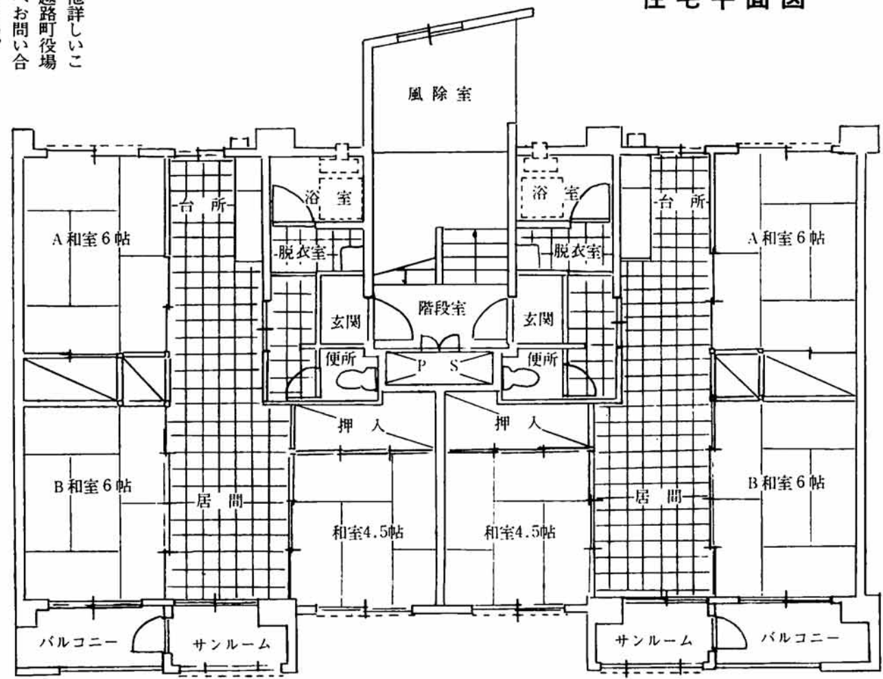
住宅平面図
