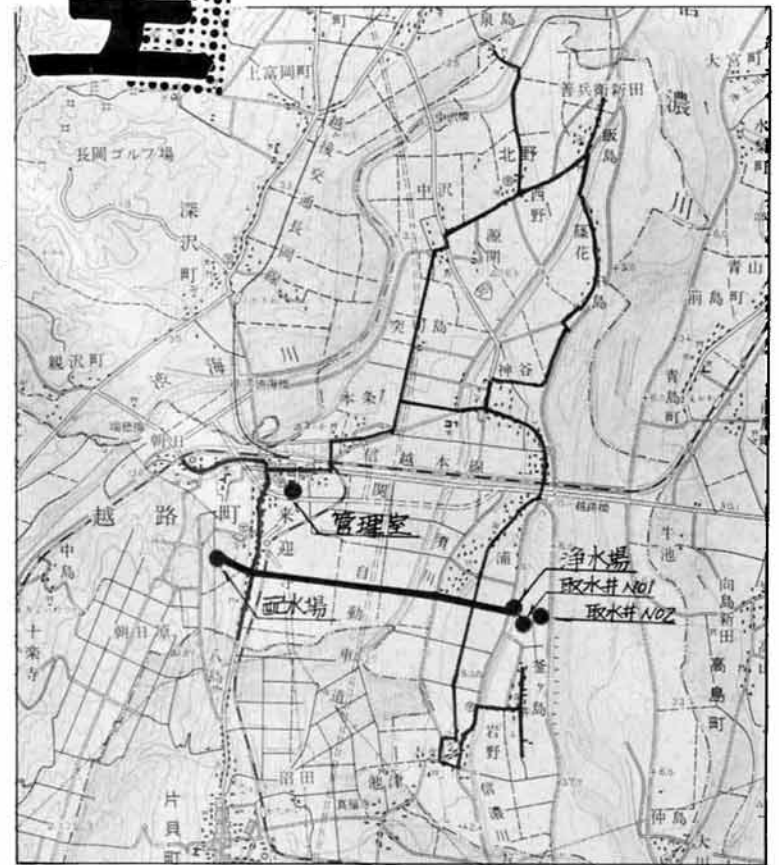
東部地区水道配管図
