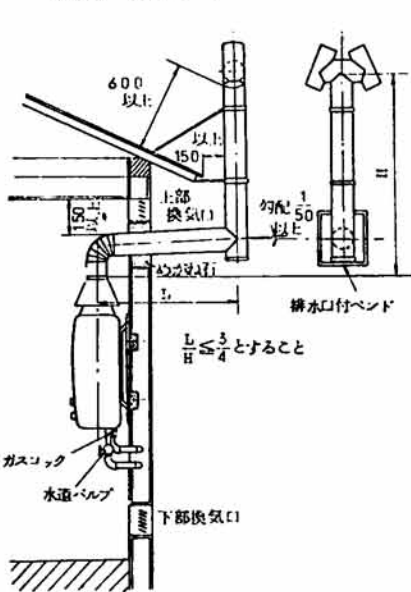
図-2 湯沸器の排気筒
