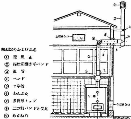
図-1 風呂の排気筒
