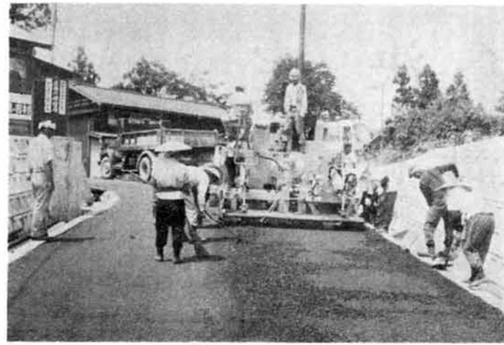
フェニッシャーによりアスファルトを布設します
