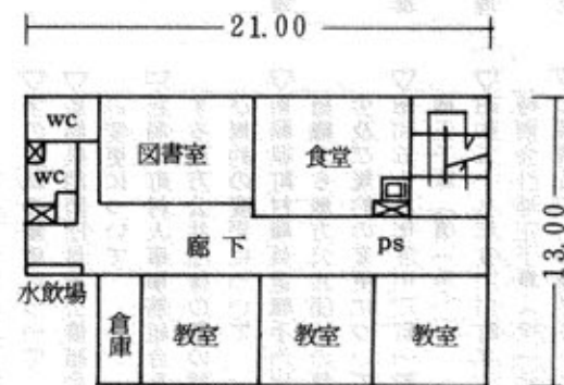
2階 平面図
