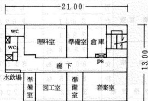
3階 平面図
