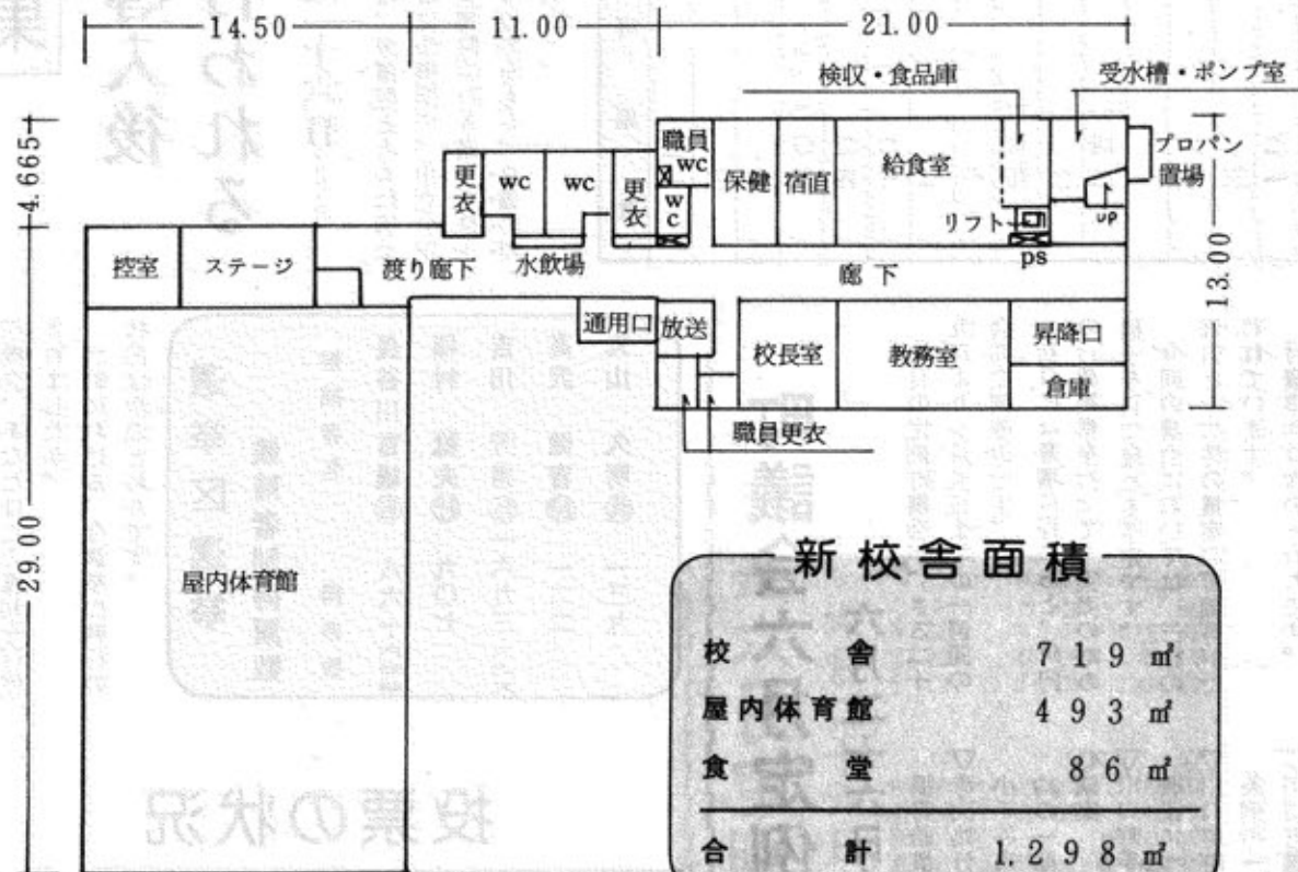
1階 平面図
