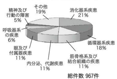
H20年5月疾病別件数
