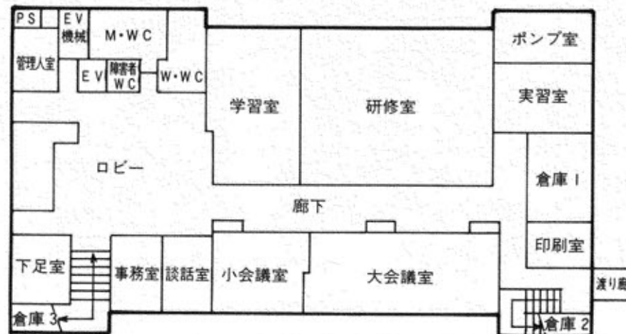
1階平面図
